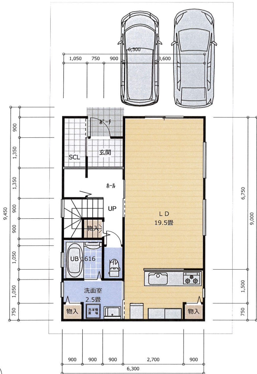
1階 縮尺 1/100
